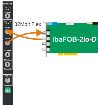
ibaLink-VME
